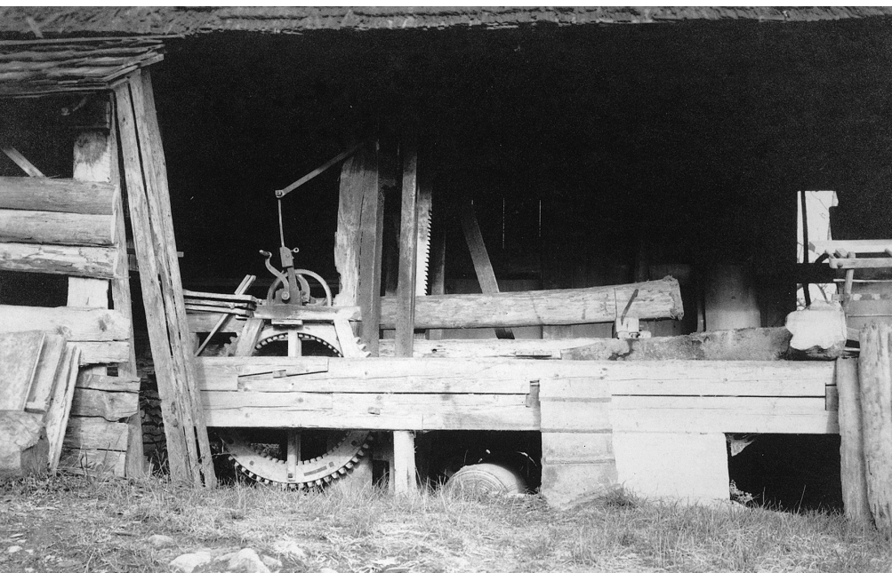
Einblick in alte Säge am Wissibächli im Kleinteil
